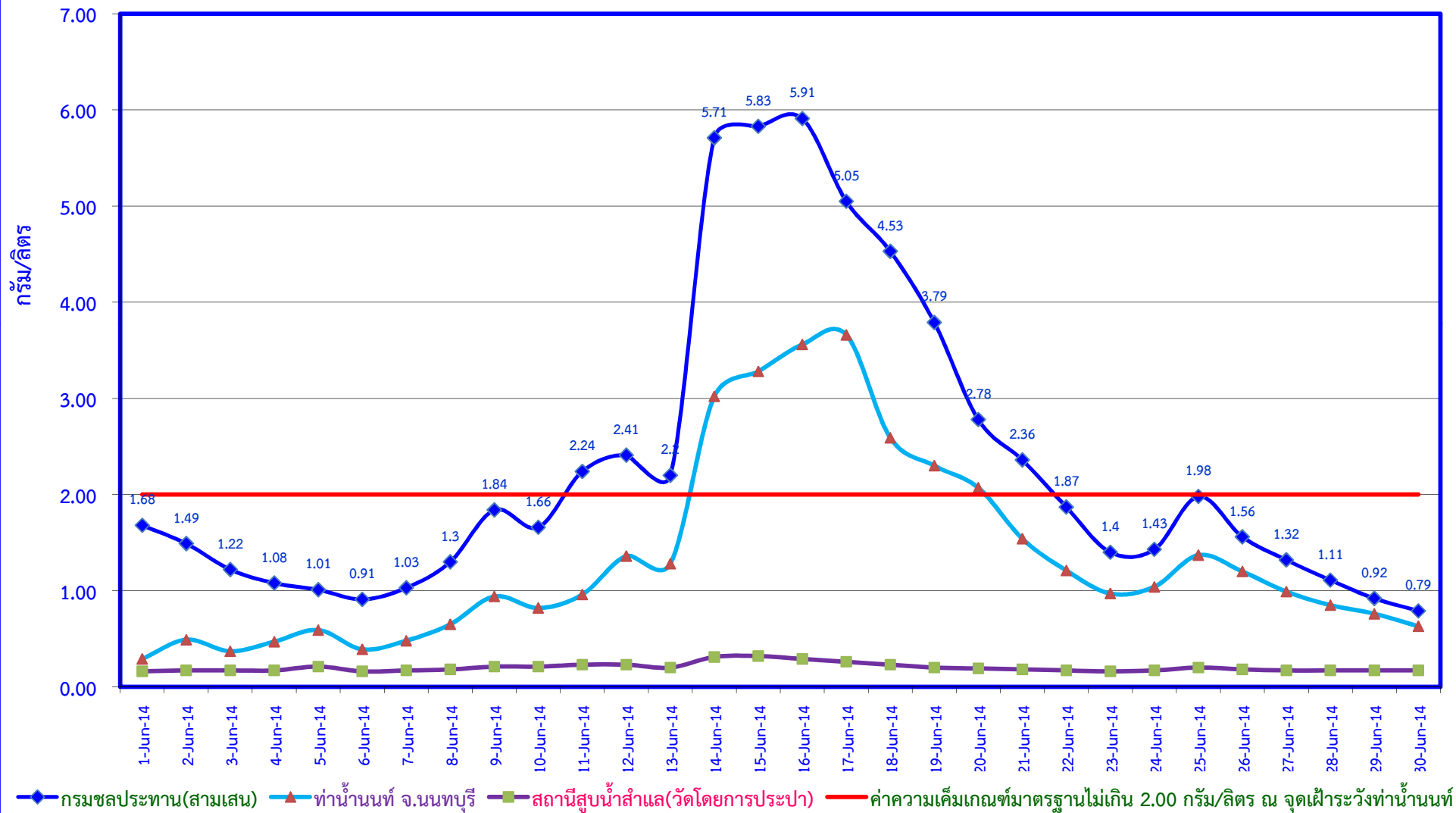
ค่าความเค็มแม่น้ำเจ้าพระยาที่กรมชลประทาน(สามเสน) ทำน่านนท์ และสถานีสูบน้ำประปาสำแล ประจำเดือนมิถุนายน ปี 2557
